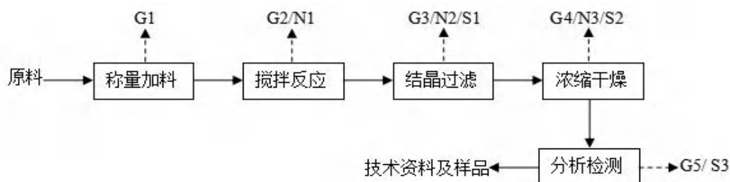
图 4-2 项目保健品原材料研发实验步骤及产污环节图
